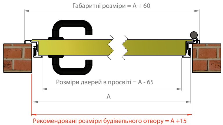
Переріз A-A
